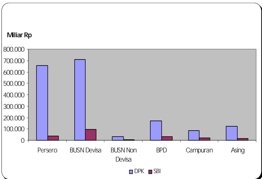
Grafik 2. Dana Pihak Ketiga dan SBI Kelompok Bank April 2009
