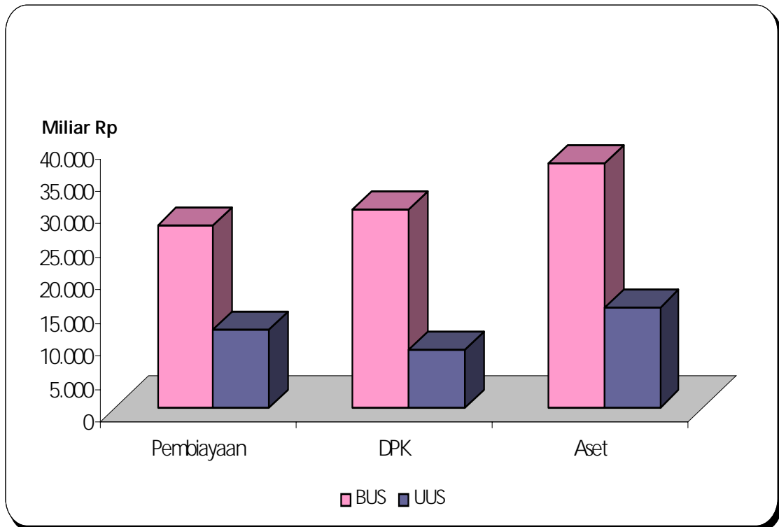
Grafik 4. Pembiayaan, DPK dan Aset Perbankan Syariah April 2009
